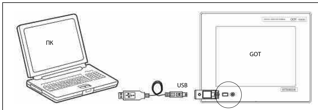
Рис. 6: Схема подключения
