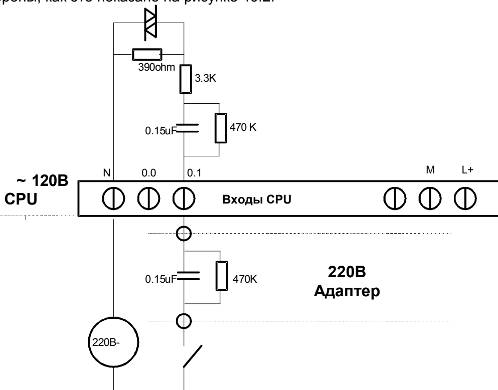
Рис 40.2: ~220В Адаптер
