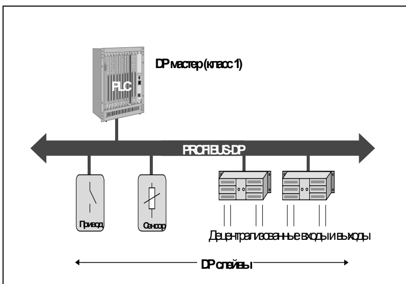
Рисунок 2: PROFIBUS-DP система
