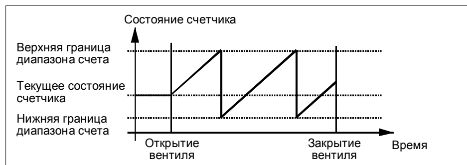
Рис. 9-1. Бесконечный счет с вентильной функцией
