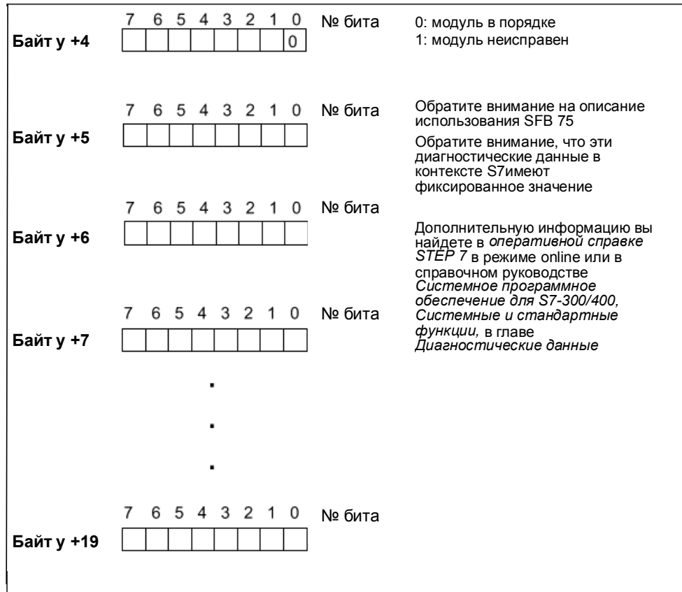
Рис. 11-11. Байты с u+4 по u+7 для диагностического прерывания (SFB 75)
