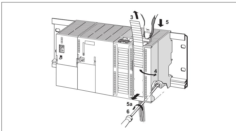
Рис. 10-1. Деблокировка фронтштекера и демонтаж модуля
