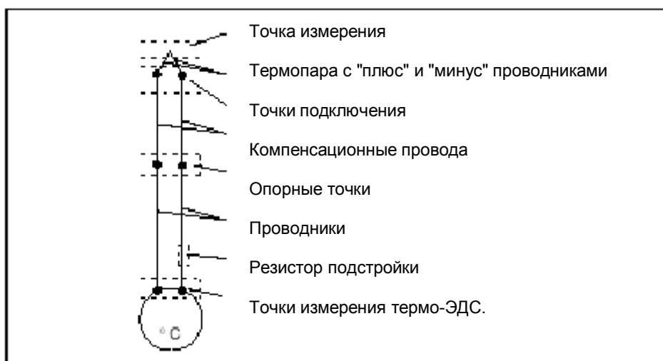
Рис. 10-3 Конструкция термоэлементов
