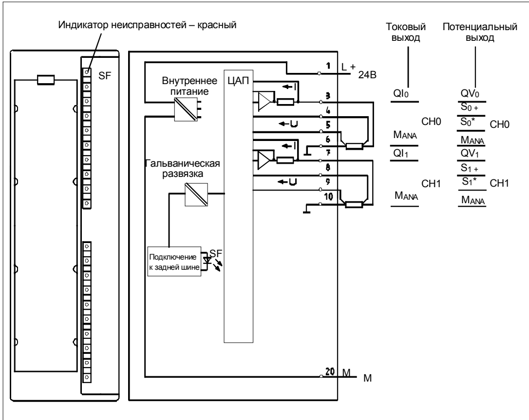
Рис. 4–35. Внешний вид и принципиальная схема аналогового модуля вывода SM 332; AO 2 × 12 Bit
