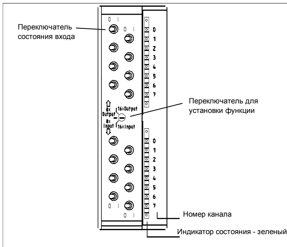
Рис. 5–1. Внешний вид имитатора SM 374; IN/OUT 16
